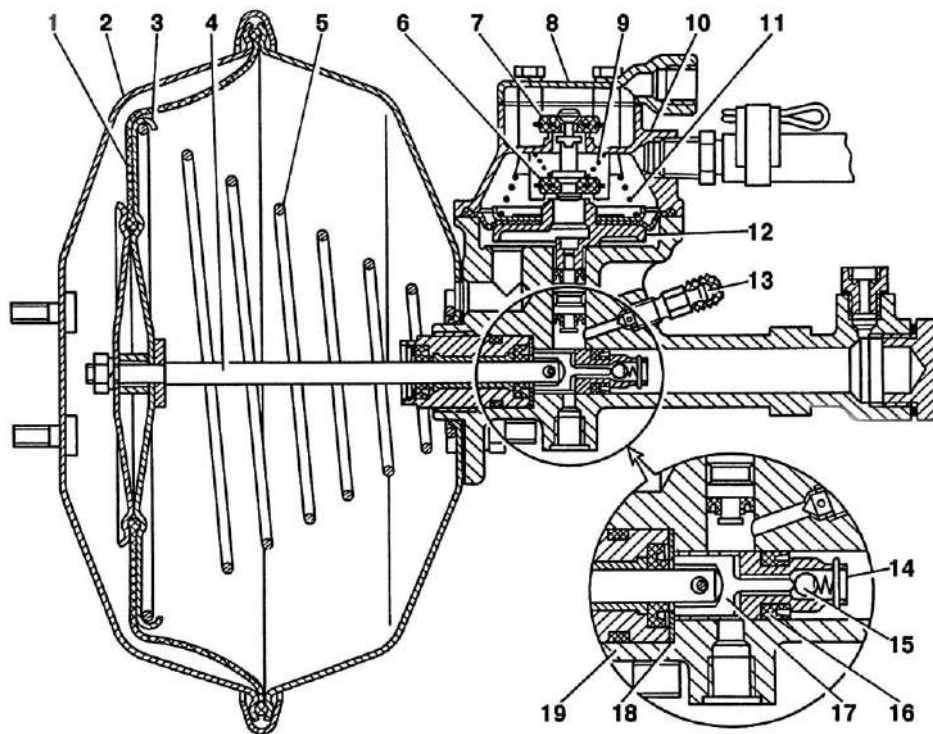
Рис. 6.17 Гидровакуумный усилитель
