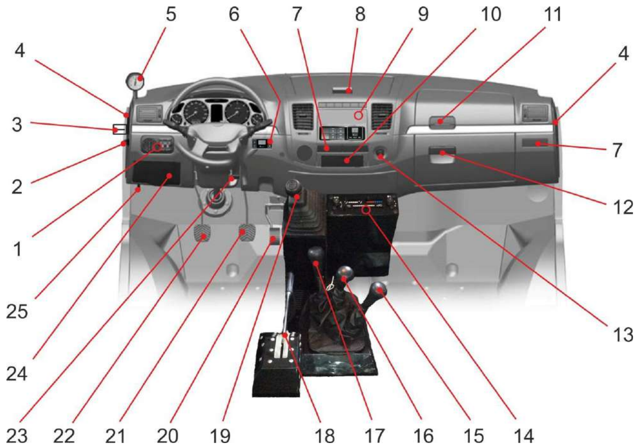
Рис. 5.6 Органы управления:
