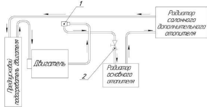
Рис. 6.20. Система отопления:
